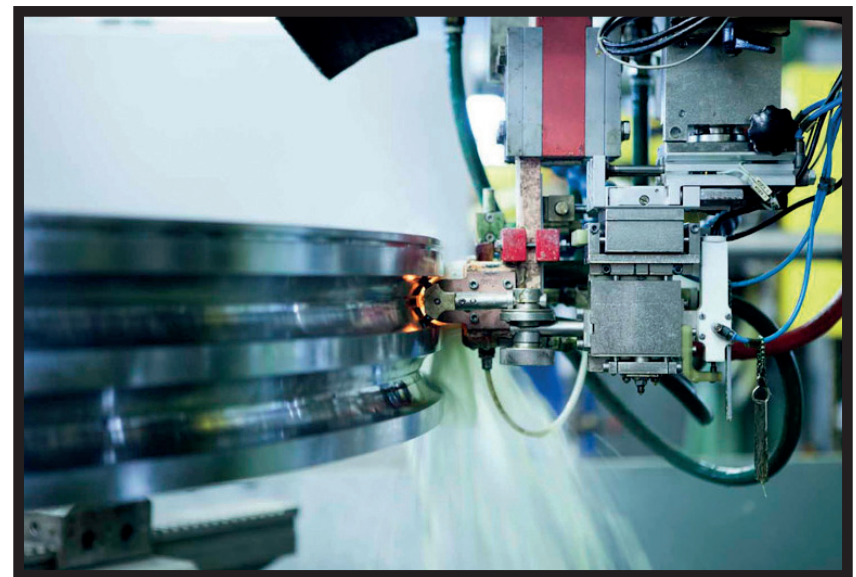
Härdning av kul- & rullagerbana
