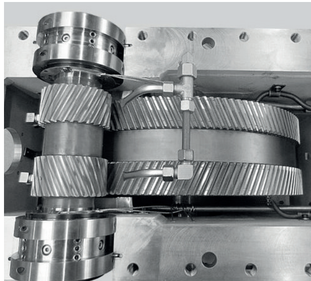
Renovering av turboväxellåda till Vattenfall.
