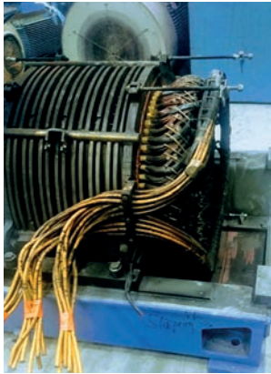
Omlindning av stator och rotor samt ny magnetplåt för släpningad motor 500 kW, LKAB.
