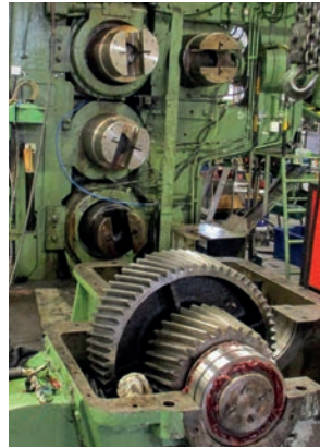
Renovering av kuggväxel till gummikalander, Trelleborgs Industri.
